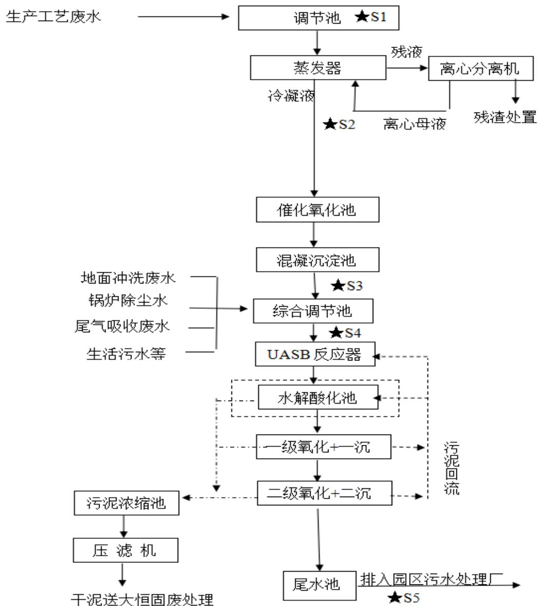
图 4.3-17 污水处理工艺图
