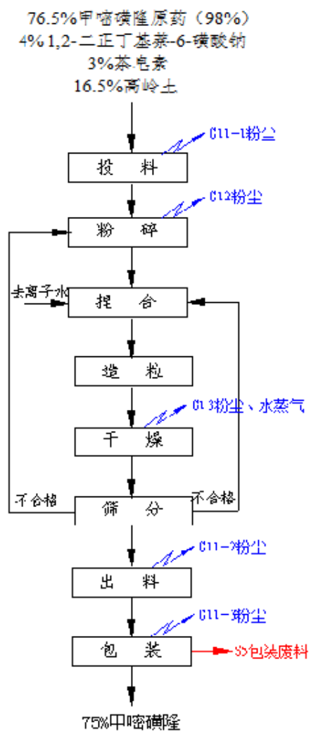
图 4.3-15 甲噁磺隆生产工艺流程图
