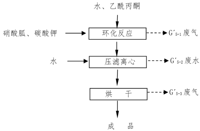
图 4.3-7 SMM 生产工艺流程图
