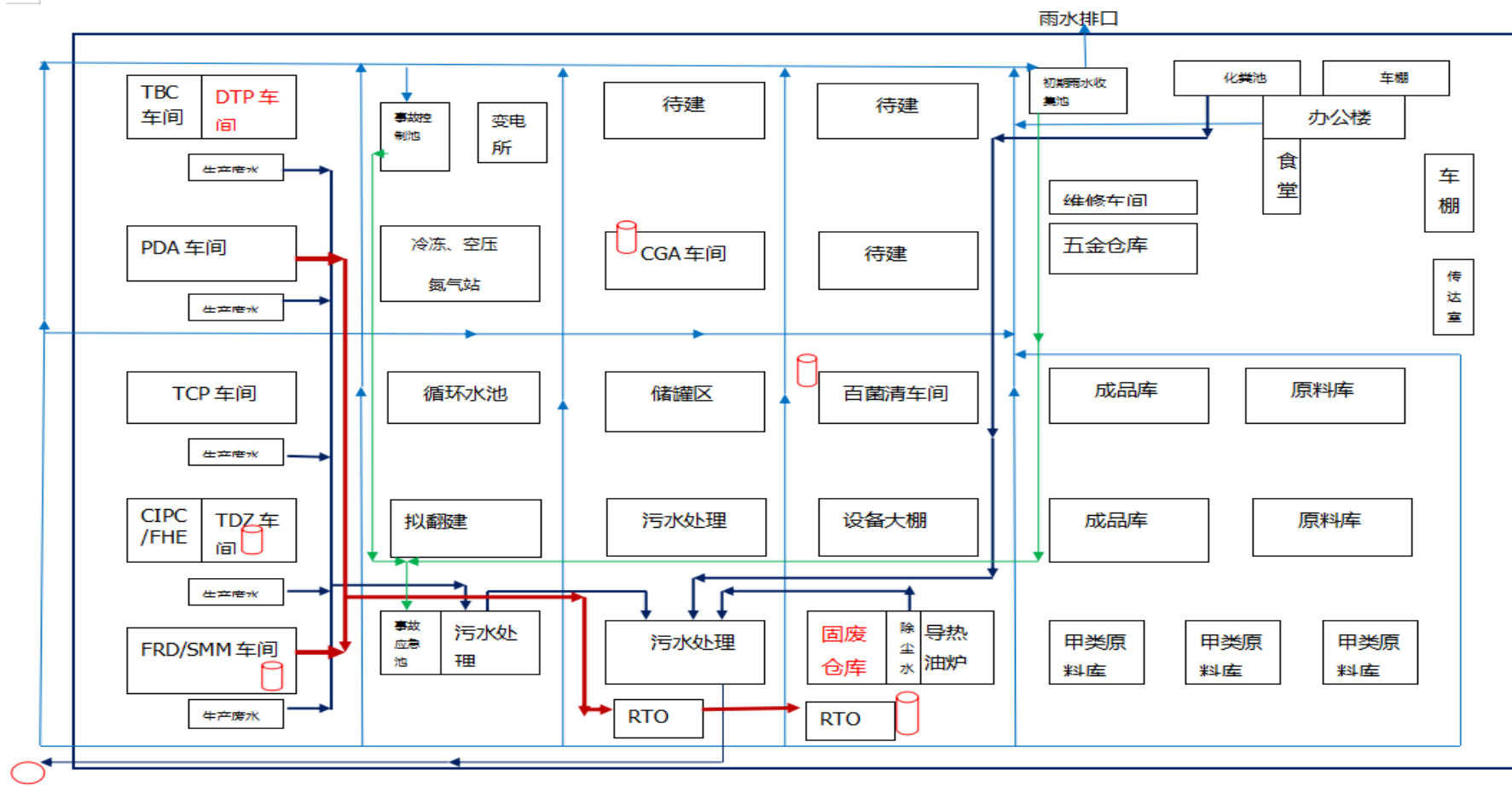
迈克斯（如东）化工有限公司东厂区雨水、废水、废气管网示意图
